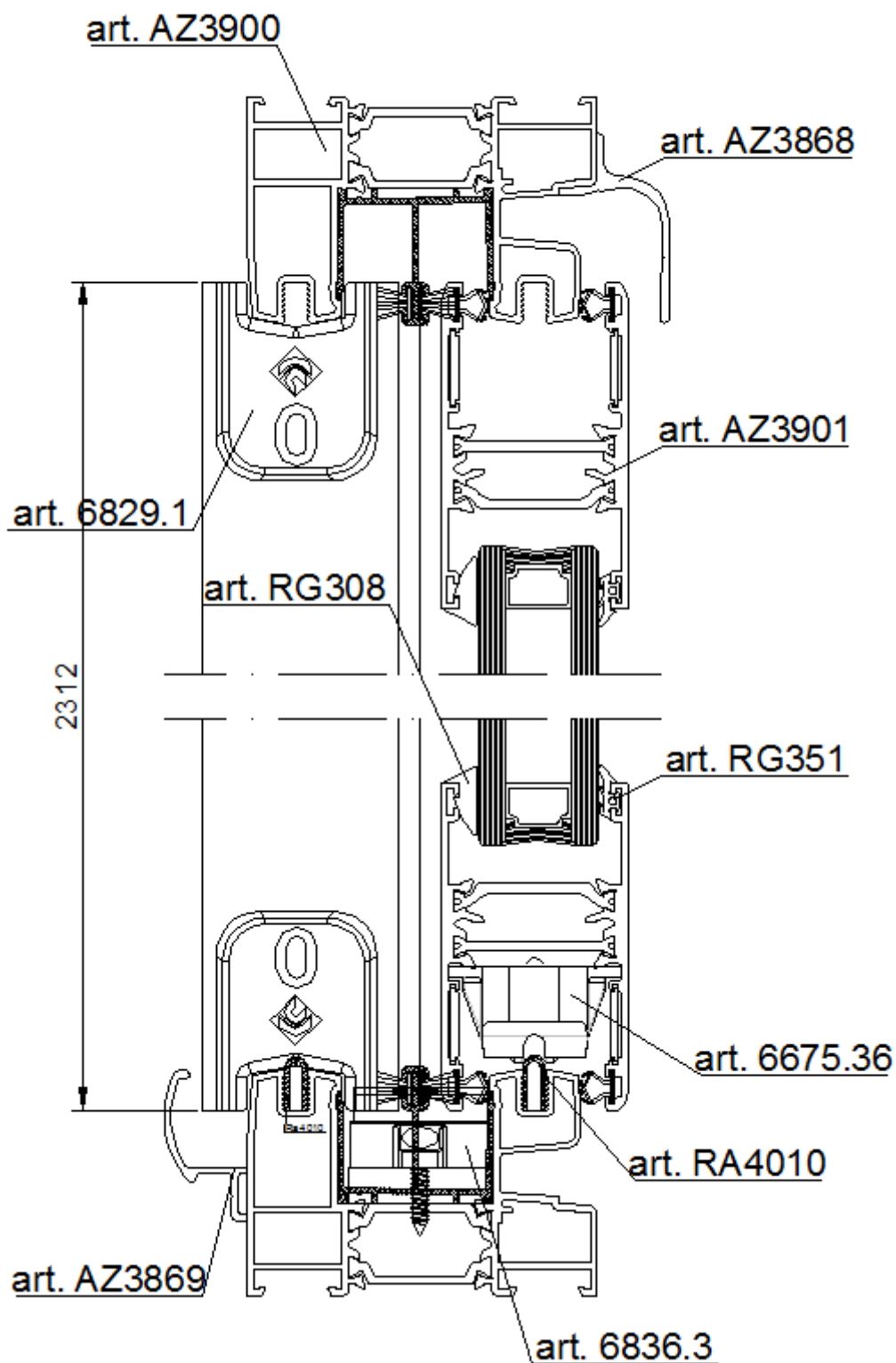
Fig. 3. Sezione B-B del campione sottoposto a prova (dimensioni nominali dichiarate, espresse in mm)
