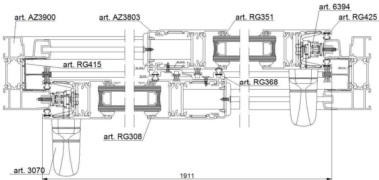
Fig. 2. Sezione A-A del campione sottoposto a prova (dimensioni nominali dichiarate, espresse in mm)
