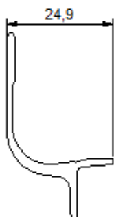
Profilato gocciolatoio art. AZ3868
