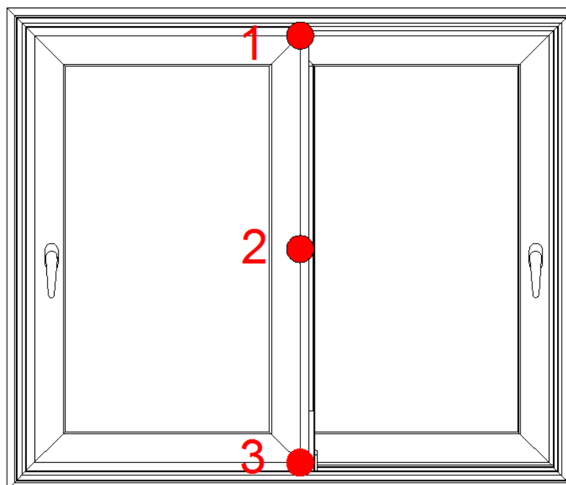
Fig. 8. Assetto sperimentale prova di resistenza al carico del vento: schema di posizionamento dei trasduttori (vista interna)
