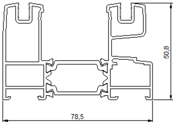
Profilato gocciolatoio art. AZ3868
